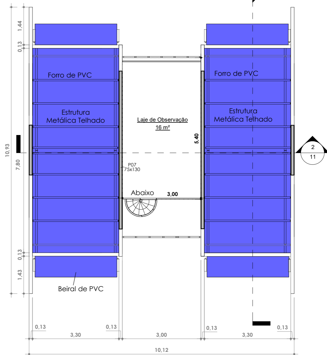
2 Laje de Observação Construir 1 : 75
