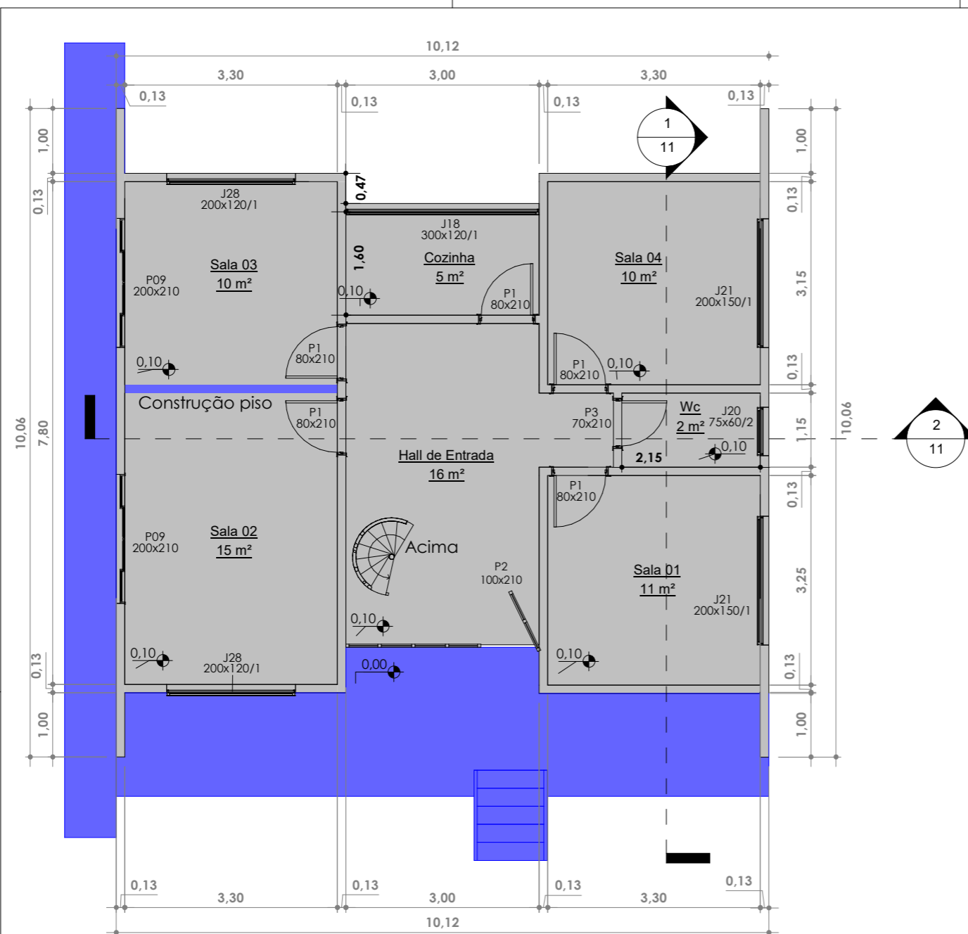
1 Térreo Construir 1 : 75
