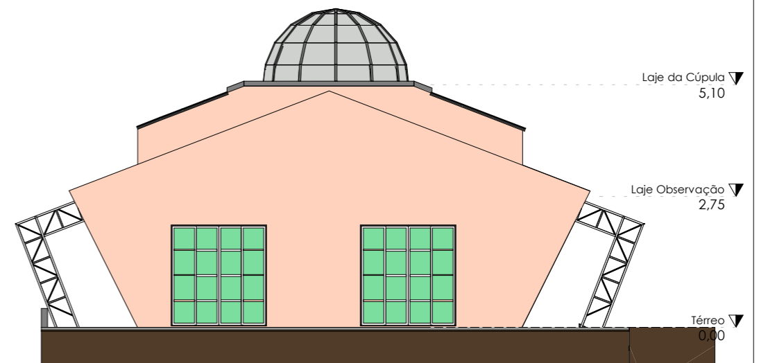
3 Elevação Oeste- Projeto Final 1 : 100
