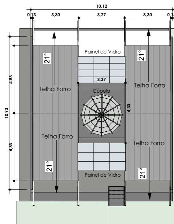
3 Implantação e Cobertura 1 : 150
