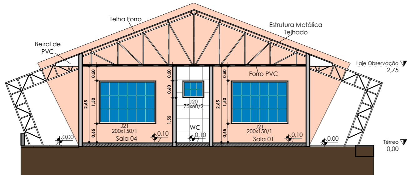
1 Corte 1 - Projeto Final 1 : 75
