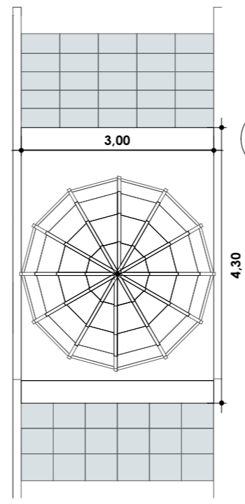
2 Laje, Cúpula e Paineis de Vidro 1 : 75
