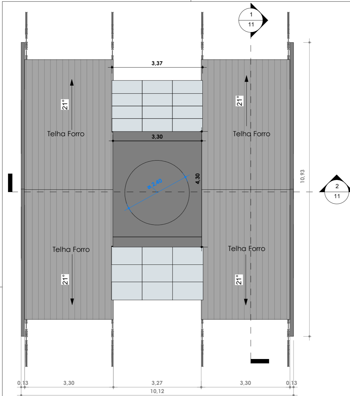
1 Laje da Cúpula Projeto Final 1 : 75
