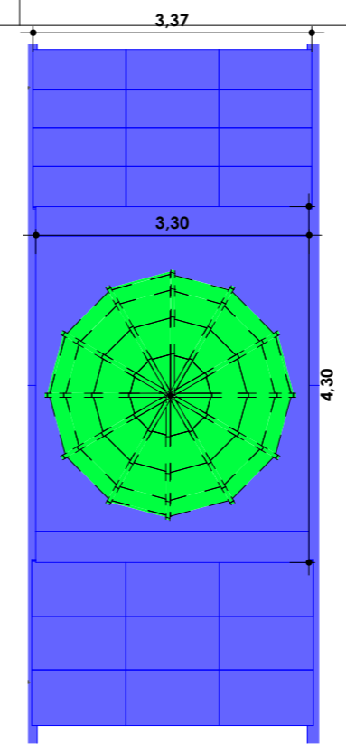
2 Laje, Cúpula e Paineis de Vidro - Construir/Recolocar 1 : 75
