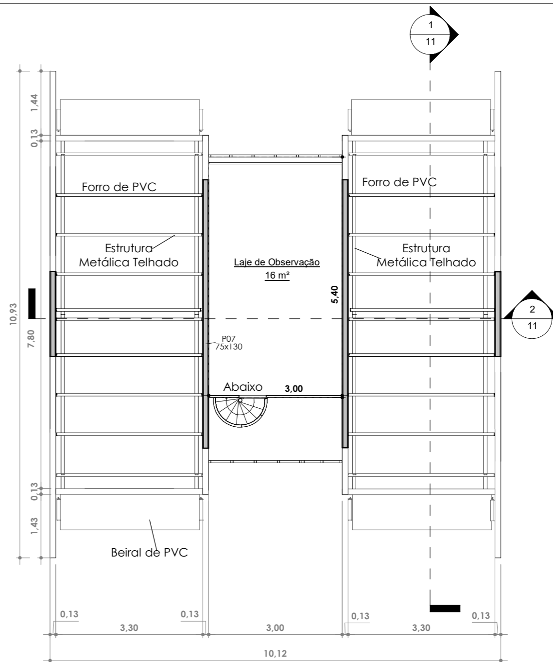
2 Laje de Observação Projeto Final 1 : 75
