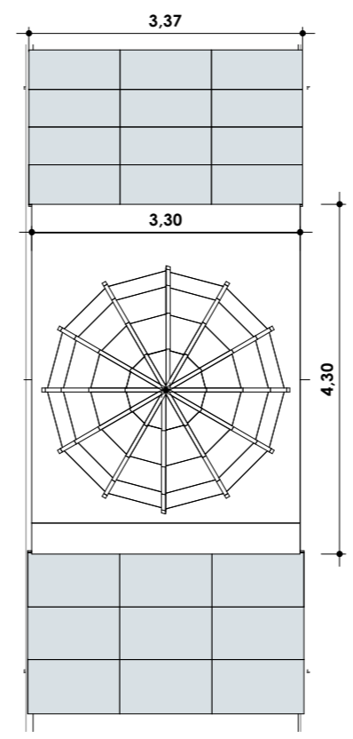
2 Laje, Cúpula e Paineis de Vidro - Projeto Final 1 : 75
