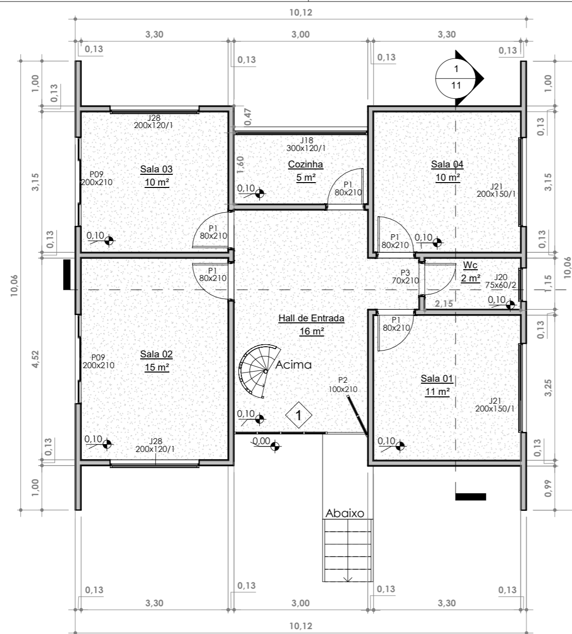
1 Térreo Existente 1 : 75
