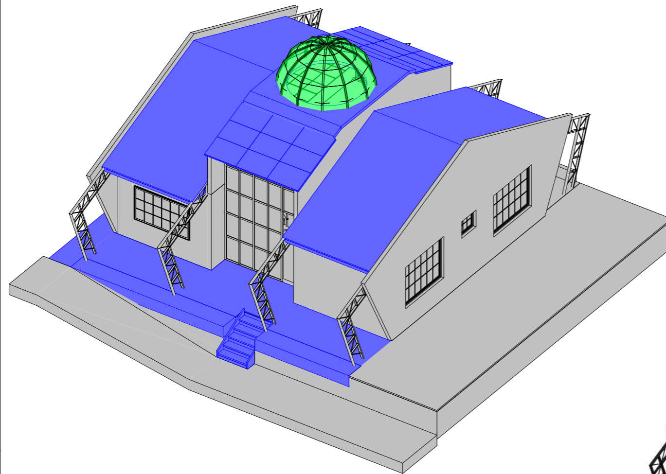
1 Perspectiva 3D Projeto Construir/Recolocar
