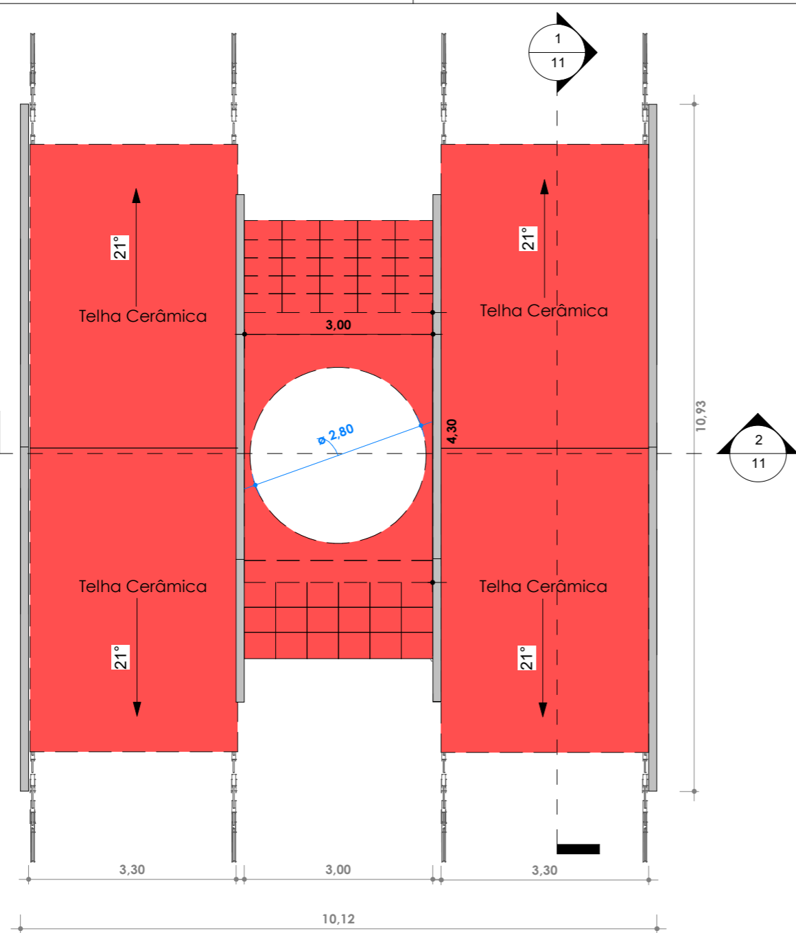
1 Laje da Cúpula Demolir 1 : 75
