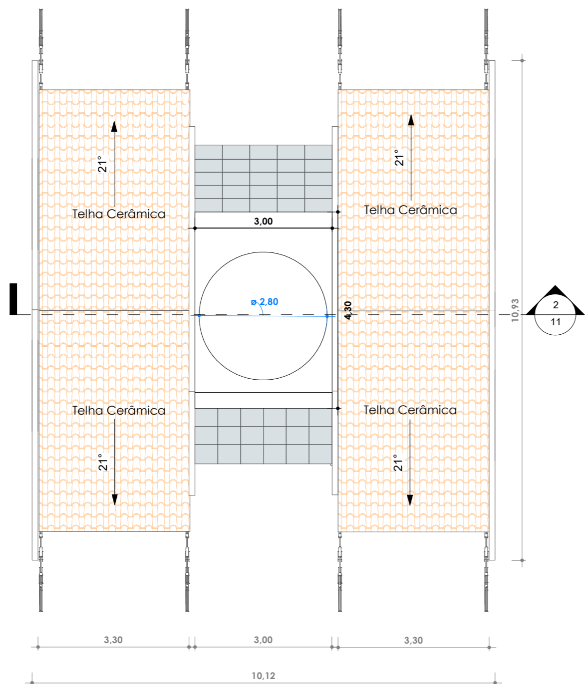
1 Laje da Cúpula Existente 1 : 75
