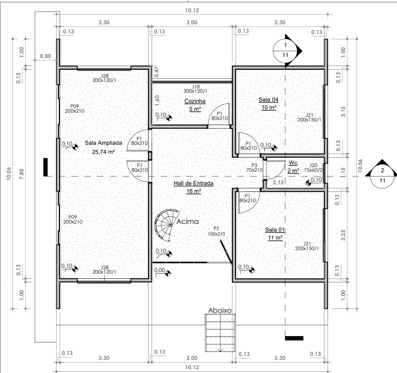
1 Térreo Projeto Final 1 : 75
