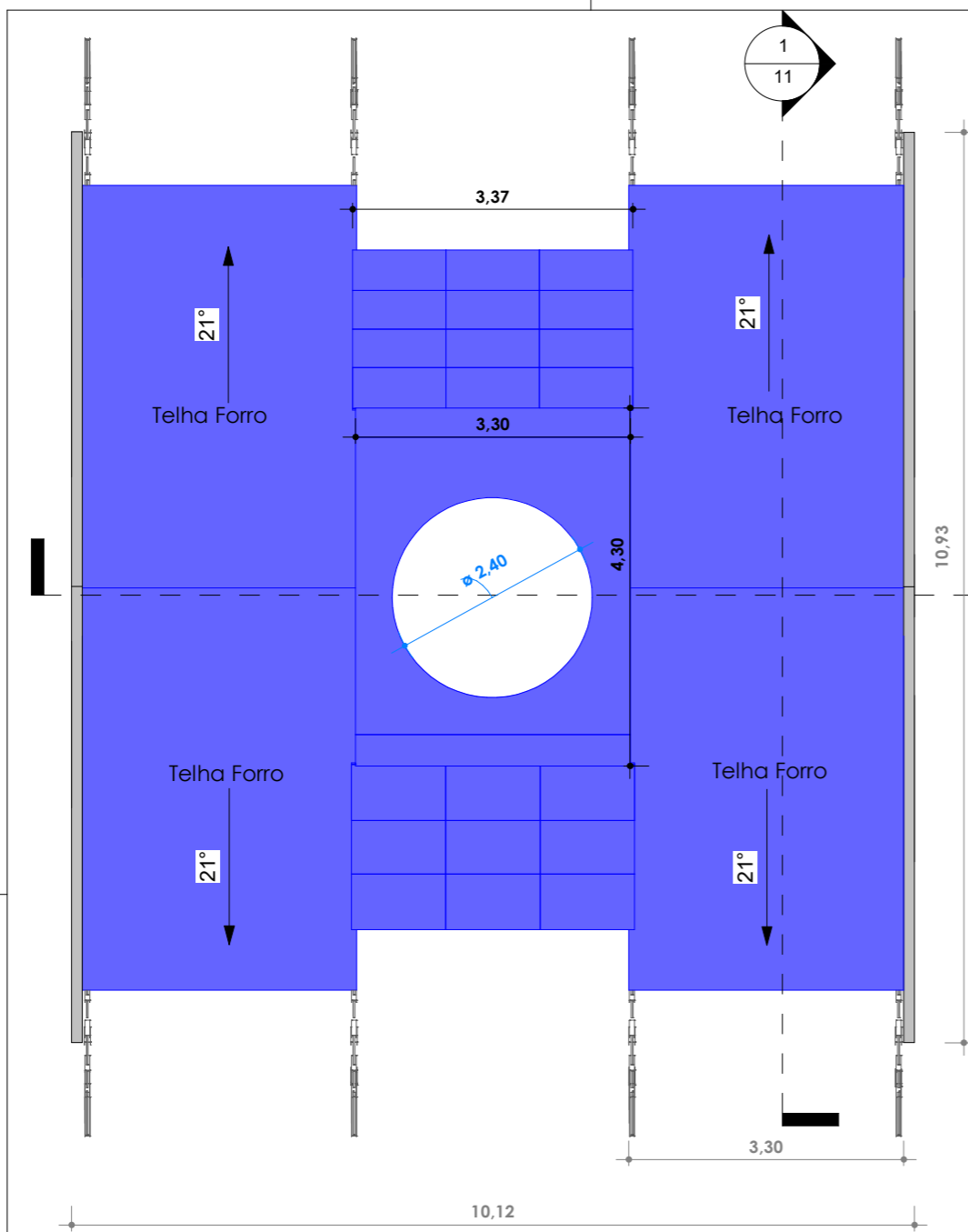
1 Laje da Cúpula Construir 1 : 75
