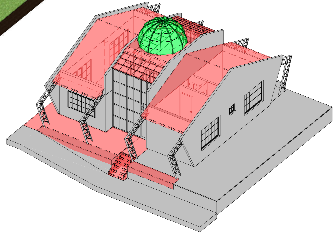
2 Perspectiva 3D Projeto Demolir/Remover
