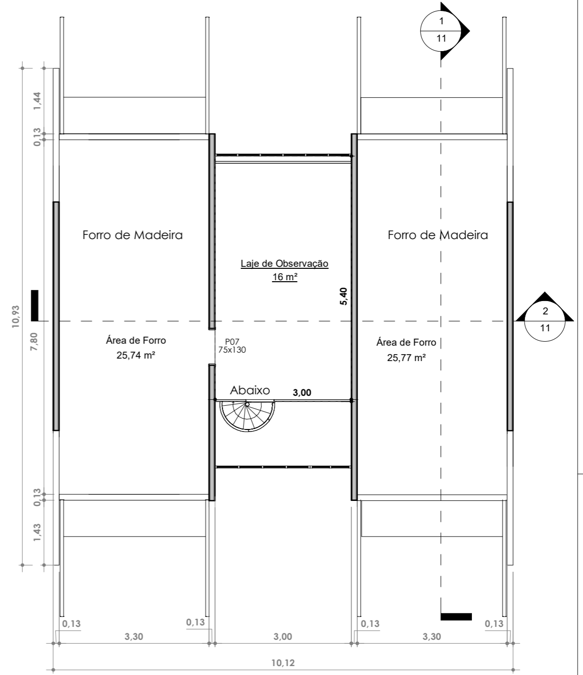
2 Laje de Observação Existente 1 : 75
