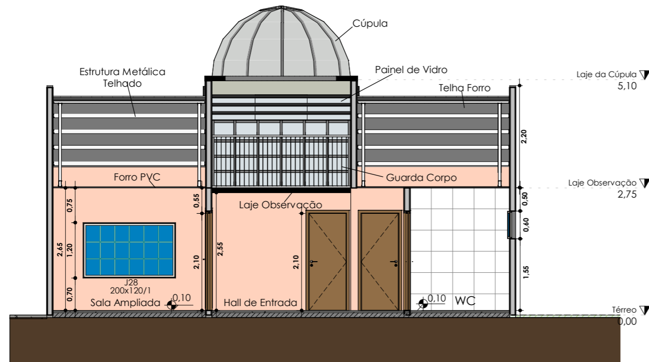
2 Corte 2 - Projeto Final 1 : 75
