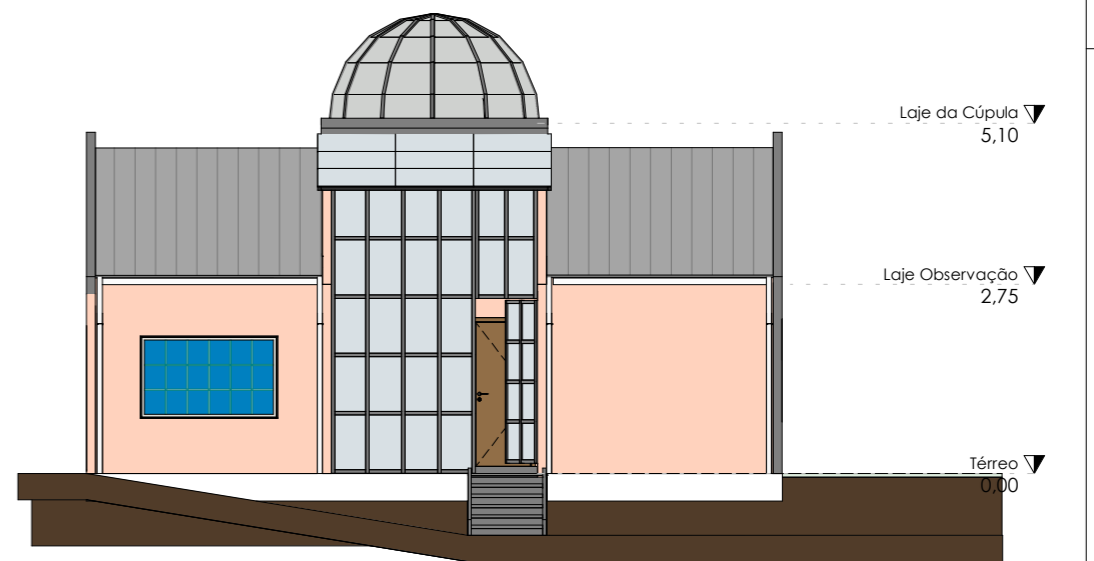
4 Elevação Sul - Projeto Final 1 : 100
