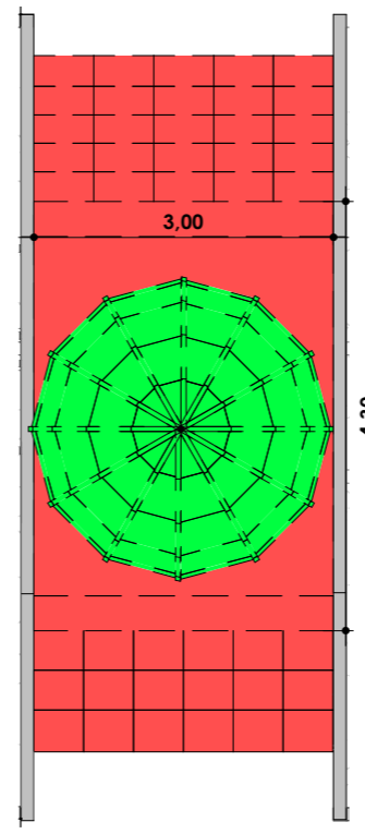
2 Laje, Cúpula e Paineis de Vidro - Demolir/Remover 1 : 75
